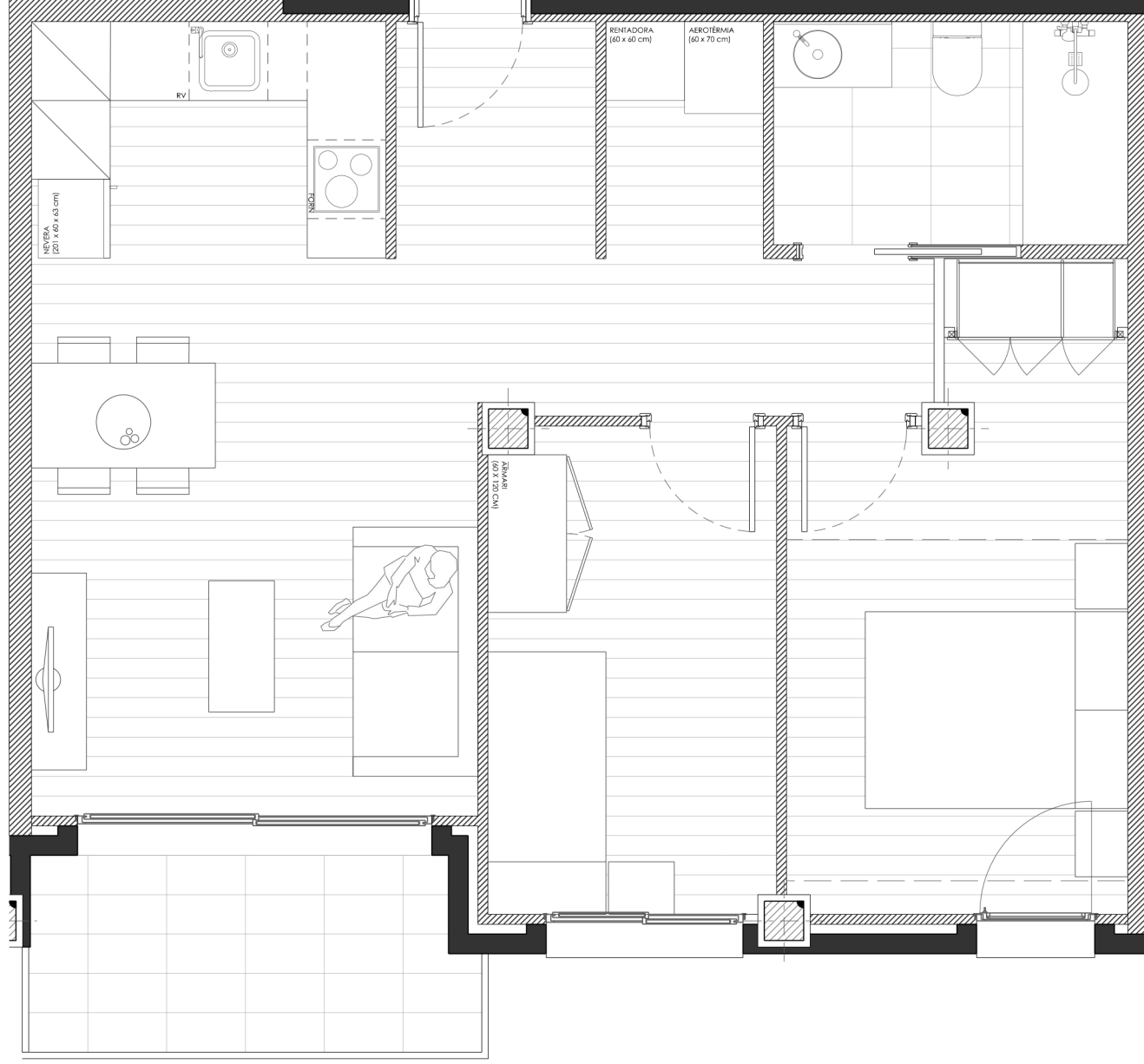
Planta Tercera - Porta 2 E. 1/50
